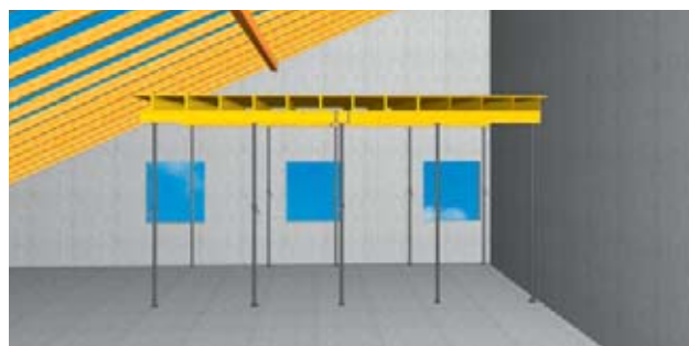
2 Ponteggio di ritenuta in fase di allestimento. Questo deve essere prolungato fino a proteggere l'intera zona a rischio di caduta.
