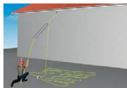
3 Sistema di lancio con fionda industriale per l'installazione del sistema di arresto caduta in caso di lavori di breve durata (vedi regola 8)
